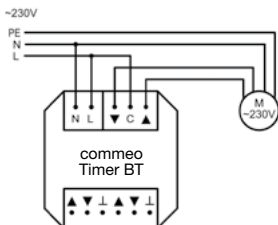
Anschluss 230-V-Antrieb
