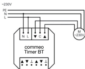
Aansluiting 230-V-aandrijving
